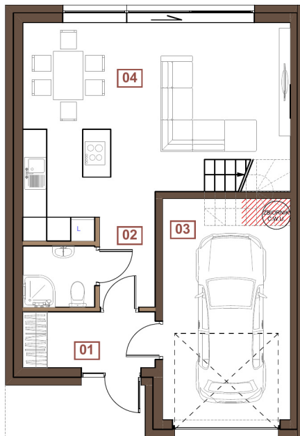
RZUT PARTERU
